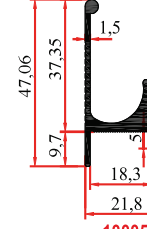
10005 0,535 Kg/m
