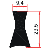
6013 E 0,515 Kg/m
