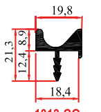
1013 ÇO 0,345 Kg/m
