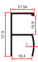
9475 0,265 Kg/m
