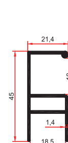
SM 1013 0,485 Kg/m
