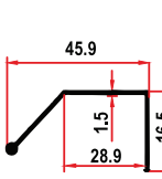
7327 BRN 0,325 Kg/m
