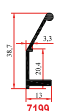
7199 0,275 Kg/m
