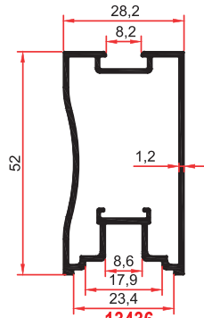
13436 0,625 Kg/m
