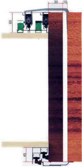
Ayarlı Dış Üst Makara
