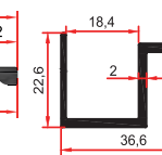
7505 0,410 Kg/m
