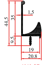
1013 ÇZ 0,520 Kg/m
