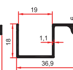
8781 0,295 Kg/m
