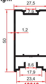
13018 0,570 Kg/m
