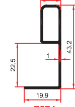
7574 0,265 Kg/m
