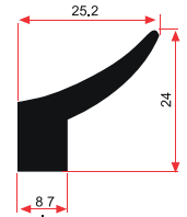
E 1656 0,520 Kg/m
