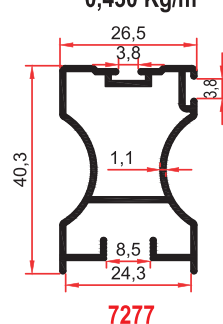
7277 0,480 Kg/m
