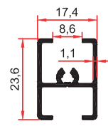
8062 0,255 Kg/m
