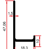
13440 A 0,305 Kg/m
