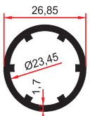
SM 5023 0,415 Kg/m
