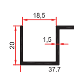
9435 0,335 Kg/m
