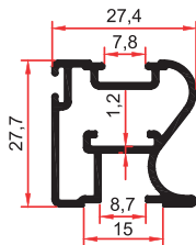
7345 0,470 Kg/m
