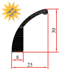
PRF-30165 0,465 Kg/m
