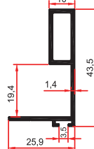
6622 0,405 Kg/m
