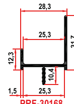
PRF-30168 0,320 Kg/m
