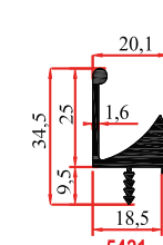
5421 0,485 Kg/m
