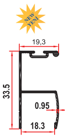
PRF-30524 0,245 Kg/m
