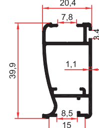
7347 0,430 Kg/m
