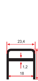
SM 1012 0,410 Kg/m
