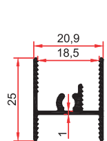
7475 0,245 Kg/m
