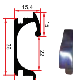
E 1228 0,390 Kg/m
