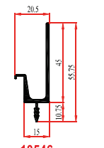
10546 0,410 Kg/m
