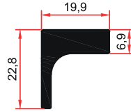
E 1304 0,510 Kg/m
