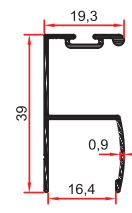
3797 A 0,255 Kg/m
