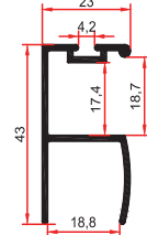
1013 BJ 0,435 Kg/m
