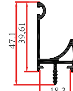
8580 A 0,510 Kg/m
