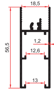
7474 0,530 Kg/m
