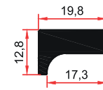
E 1092 0,420 Kg/m
