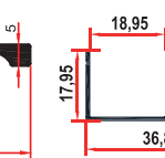
7505 EKO 0,290 Kg/m
