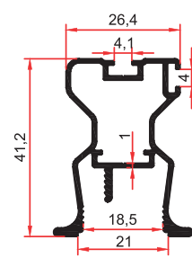
7473 0,520 Kg/m
