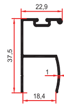
9476 0,295 Kg/m
