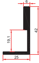
8755 0,615 Kg/m
