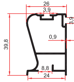
7472 0,375 Kg/m
