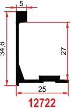
12722 0,305 Kg/m
