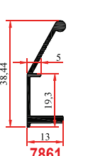
7861 0,255 Kg/m
