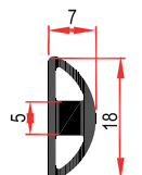
PRF-30326 0,180 Kg/m
