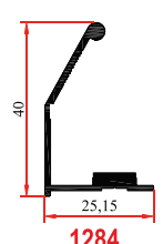
1284 0,345 Kg/m
