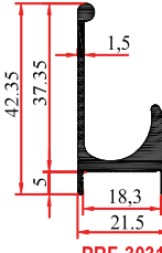
PRF-30319 0,505 Kg/m
