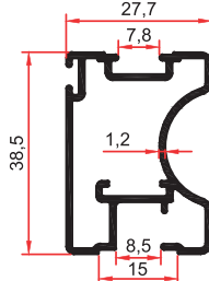
7346 0,565 Kg/m
