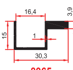
8965 0,255 Kg/m
