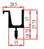
10548 0,290 Kg/m
