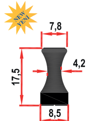
PRF-30327 0,300 Kg/m
