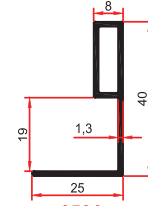
6536 0,335 Kg/m
