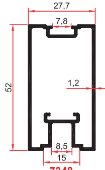
7348 0,645 Kg/m
