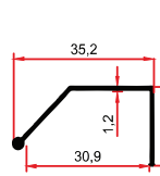
7490 0,190 Kg/m
