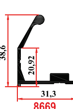
8669 0,455 Kg/m
