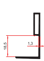
8800 0,305 Kg/m
