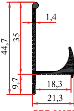
PRF-30370 0,360 Kg/m
