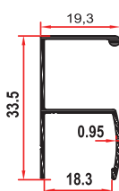
PRF-30523 0,225 Kg/m
