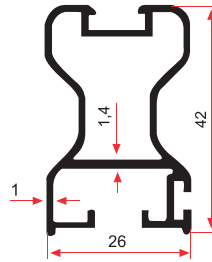
5804 0,495 Kg/m
