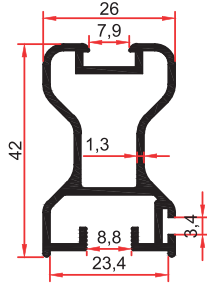
4418 0,600 Kg/m
