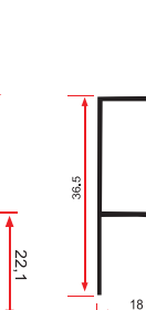
E 1910 0,225 Kg/m
