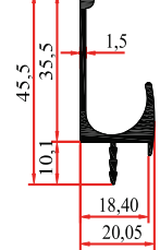
8227 0,420 Kg/m
