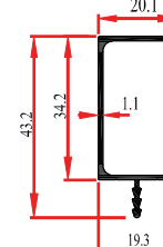
PRF-30446 0,280 Kg/m
