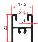
6830 0,265 Kg/m
