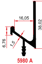
5980 A 0,410 Kg/m
