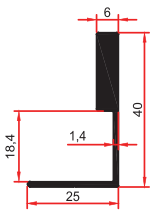
7503 0,485 Kg/m
