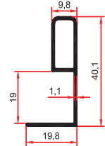
8780 0,275 Kg/m
