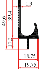
1012 ÇD 0,495 Kg/m
