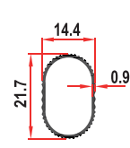
12050 0,120 Kg/m
